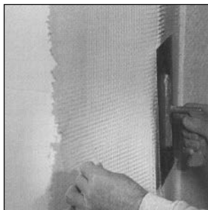
Die Dämmplatten werden nun bis zum offenen Systemende über das vorgelegte Gewebe aufgeklebt. Der Klebeflächenanteil (Kontaktfläche) von \geq 70\% ist dabei unbedingt einzuhalten.
