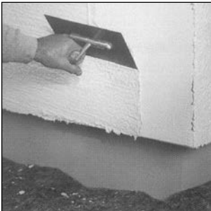
Aufziehen des Deckputzes.
