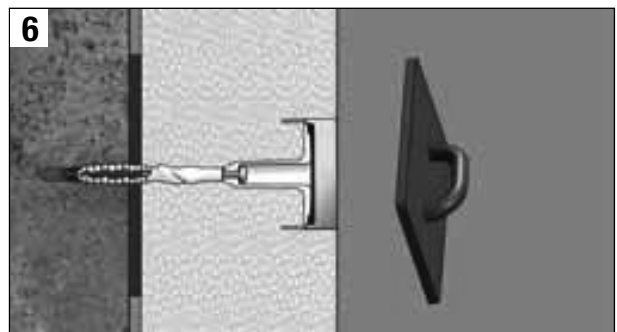
ejothem STR-Rondells einsetzen und mit einem Reibebrett oberflächenbündig eindrücken
