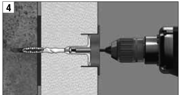
vertiefte Montage mit STR-tool
