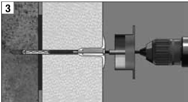
vertiefte Montage mit STR-tool
