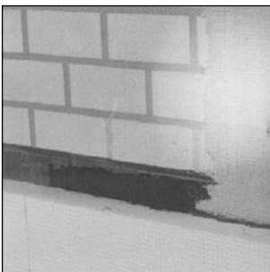
Am offenen Systemende wird ca. 20 cm breit Klebemörtel auf den Untergrund vorgelegt, in den das Dennert-Armierungsgewebe eingebettet wird. Zum freien Rand steht das Gewebe um weitere 20 cm plus der Dämmplattendicke über.
