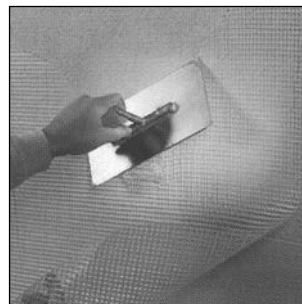
Nach dem Verkleben der Dämmplatten wird das Dennert-Armierungsgewebe an der Dämmplattenstirnseite und auf der Dämmplattenfläche in den Armierungsmörtel eingebettet. Anschließend wird das System verputzt.
