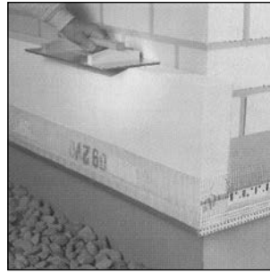
Durchschleifen der ersten Plattenreihe zur „Flucht“.
