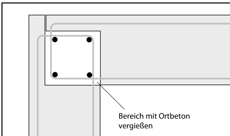
Eckausführung biegesteif
