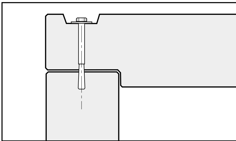
Eckausführung L-Stoß
