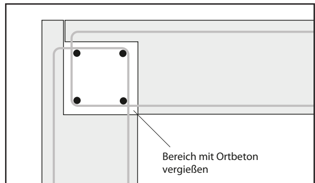
Eckausführung biegesteif
