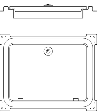
Breite Reinigungstür DIN rechts und links mit 4 Schlagdübel und Vierkant- schlüssel verzinkt und Edelstahl
